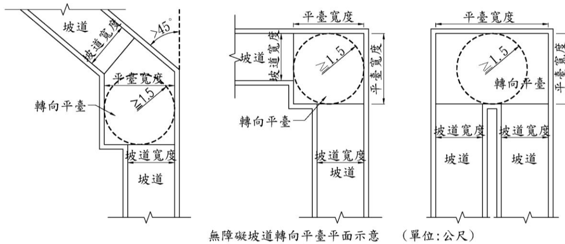
圖 14.3.1 無障礙坡道及平臺參考圖
